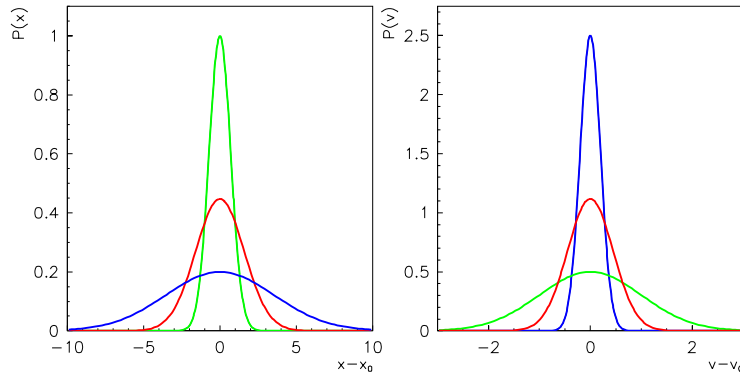
Obrázek 2: Tvar jednorozměrného vlnového balíku jako funkce prostorové souřadnice (vlevo) a rychlosti (vpravo). Tři zobrazené vlnové balíky, jejichž středy se nacházely v čase t_0 v bodě x_0 a jejichž střední rychlosti nabývaly hodnoty v_0 , se liší šířkami \Delta x ( \Delta v ) vlnových balíků v prostorové souřadnici (rychlosti). Balík, který je „úzký“ v proměnné x je „široký“ v proměnné v a naopak.
