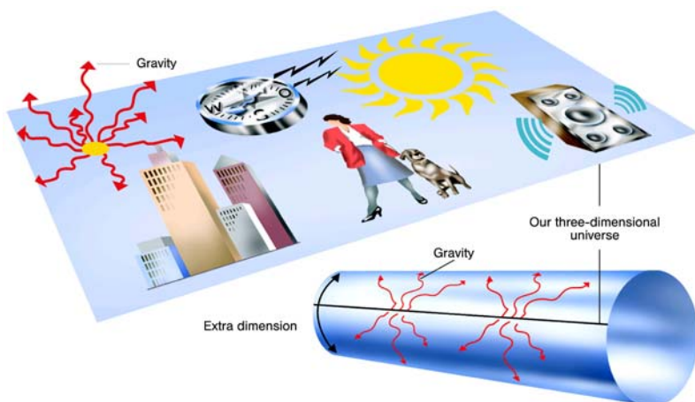
Obr. 11: Zatímco my žijeme a všechny síly kromě gravitace působí ve třírozměrném prostoru, znázorněném vodorovnou čarou na plášti válce, gravitace se šíří i ve velkých svinutých extra dimenzích, na obrázku představovaných pláštěm válce.
