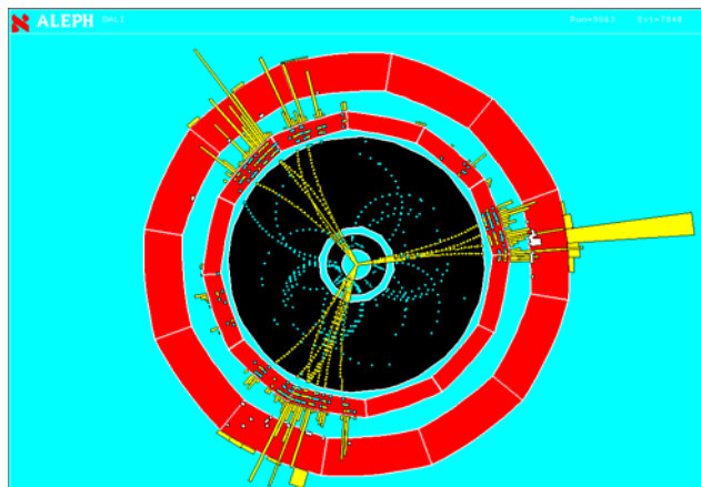
Obr. 7: Počítačová rekonstrukce výsledku srážky elektronu s pozitronem na urychlovači LEP v CERN, při níž vznikly tři jety. Energie jednotlivých částic v jetech je úměrná výšce žlutých věžiček. Obrázek je v rovině kolmé na směr srážejících se částic.
