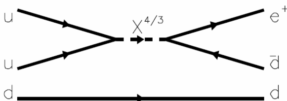
Obr. 8: Rozpad protonu v teoriích velkého sjednocení. Dvojice kvarků uu anihiluje na těžký kalibrační boson s nábojem 4/3 , jenž se poté přemění na pozitron a mezonu \pi^0 .
