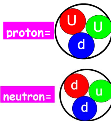
Obr. 1: kvarkové složení protonu a neutronu. V optické analogii jsou nukleony i všechny hadrony „bezbarvé“.
