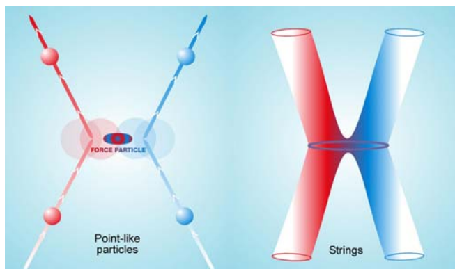
Obr. 10: Rozptyl dvou uzavřených strun ve třech rozměrech (vpravo). Na obrázku vlevo je analogický proces pro bodové částice.
