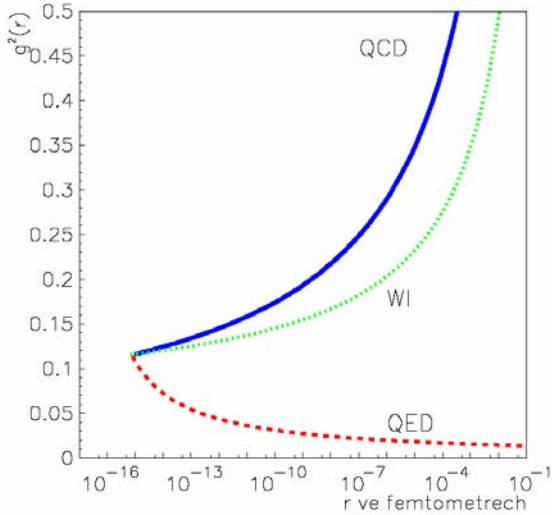
Obr. 5: závislost efektivních nábojů silných (plná čára), slabých (tečkovaná) a elektromagnetických sil (čárkovaná) na vzdálenosti.
