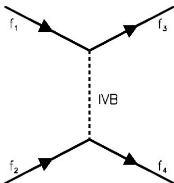
Obr. 2: Diagram znázorňující výměnný mechanismus sil mezi kvarky a leptony.
