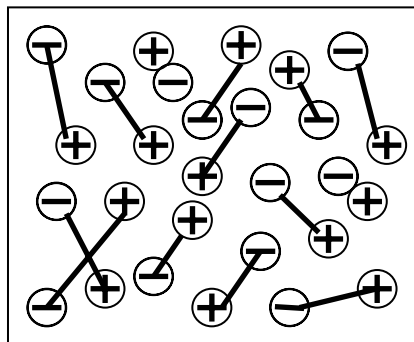
Obr. 3: Grafické znázornění vakua v QED. Virtuální elektron-pozitronové páry „žijí“ po dobu, která je úměrná délce vyznačené spojnice mezi elektronem a pozitronem.
