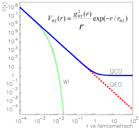
Obr. 6: srovnání závislostí elektromagnetických (čárkovaně), slabých (tečkovaně) a silných (plná čára) sil mezi dvěma kvarky či na vzdálenosti.
