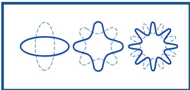
Obr. 9: Vibrační stavy jednorozměrné uzavřené struny v rovině. Vlevo základní stav s nejnižší energií, uprostřed a vpravo první dva excitované stavy.
