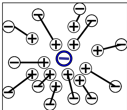
Obr. 4: Polarizace vakua v QED v důsledku vložení
